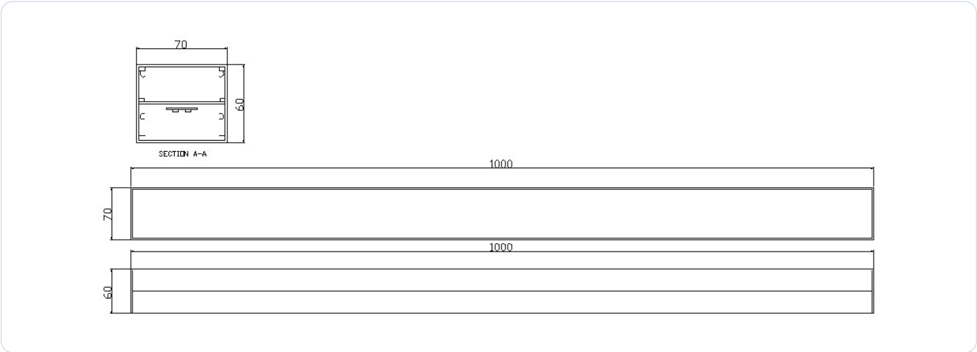
제품도면 (Unit: mm)
